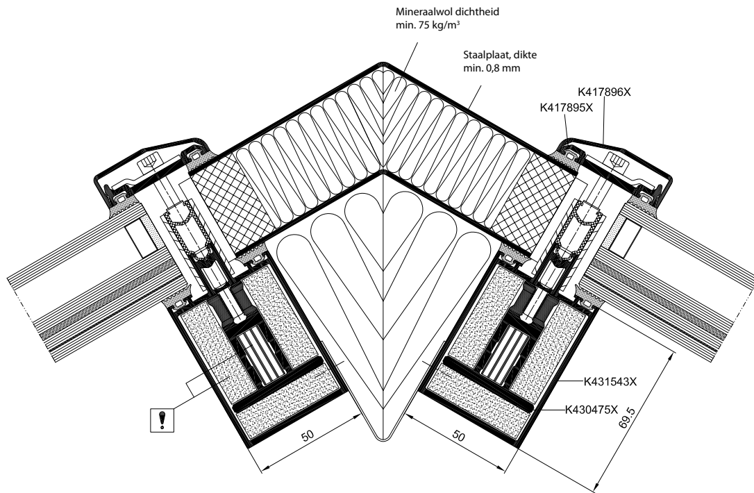
Dwarsdoorsnede door de nok van een brandwerend dak
