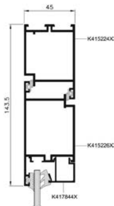
Dwarsdoorsnede deur onder zonder drempel
